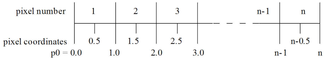
Fig. 3: Pixel coordinates
